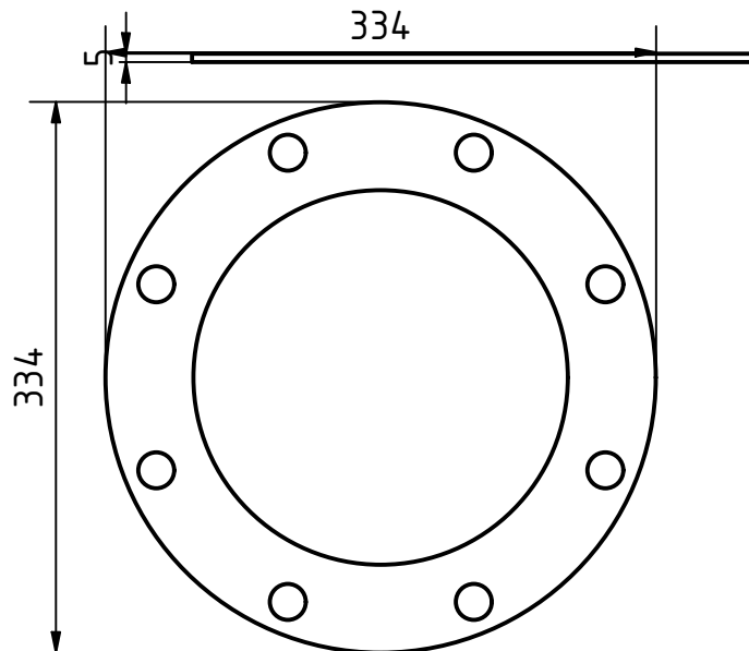
NDV-4102 Фланец трубы верхний — 1 шт. на проект
