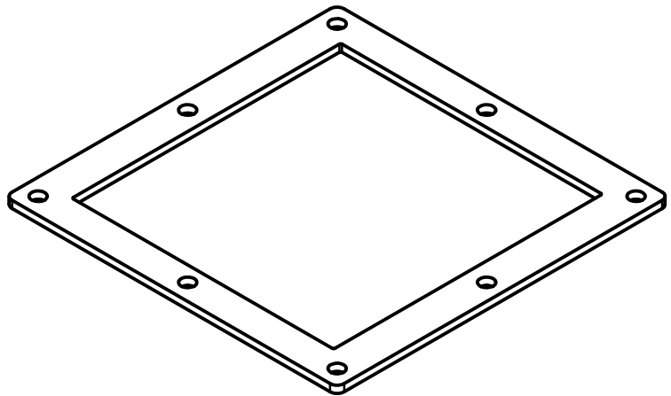
NDV-2103 Фланец коллектора, s=3.0 1 шт. на NDV-2000; 4 шт. на проект
