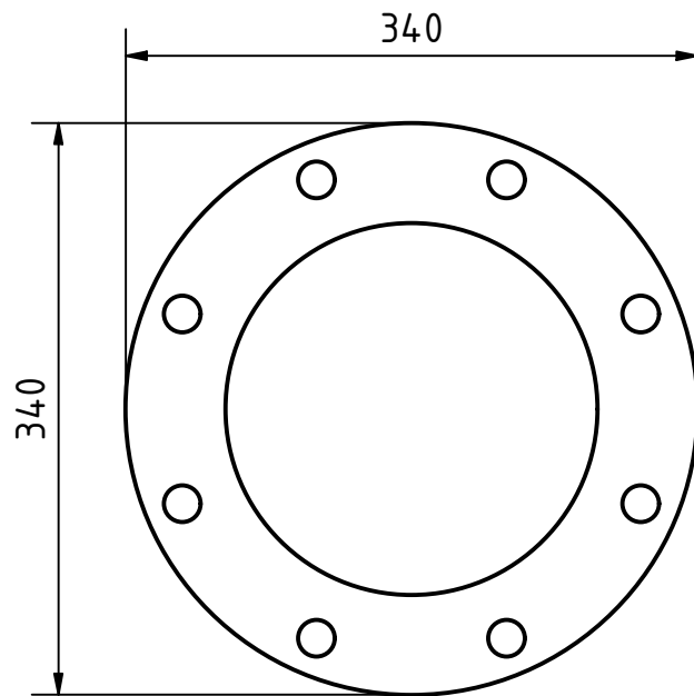
NDV-4101 Фланец трубы нижний, s=5.0
