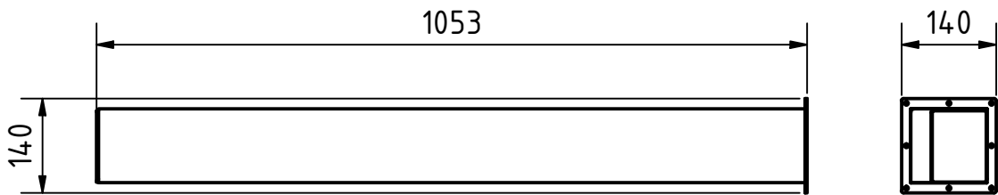
NDV-2000 Коллектор 4 шт. на проект
